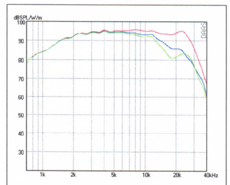
SPL VERTIKAL 0° - 5° - 15°
