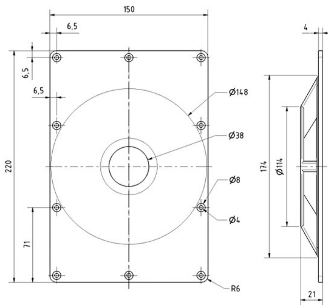
WG 220x150 01.10.10
